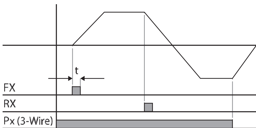
[Operacja 3-przewodowa]
