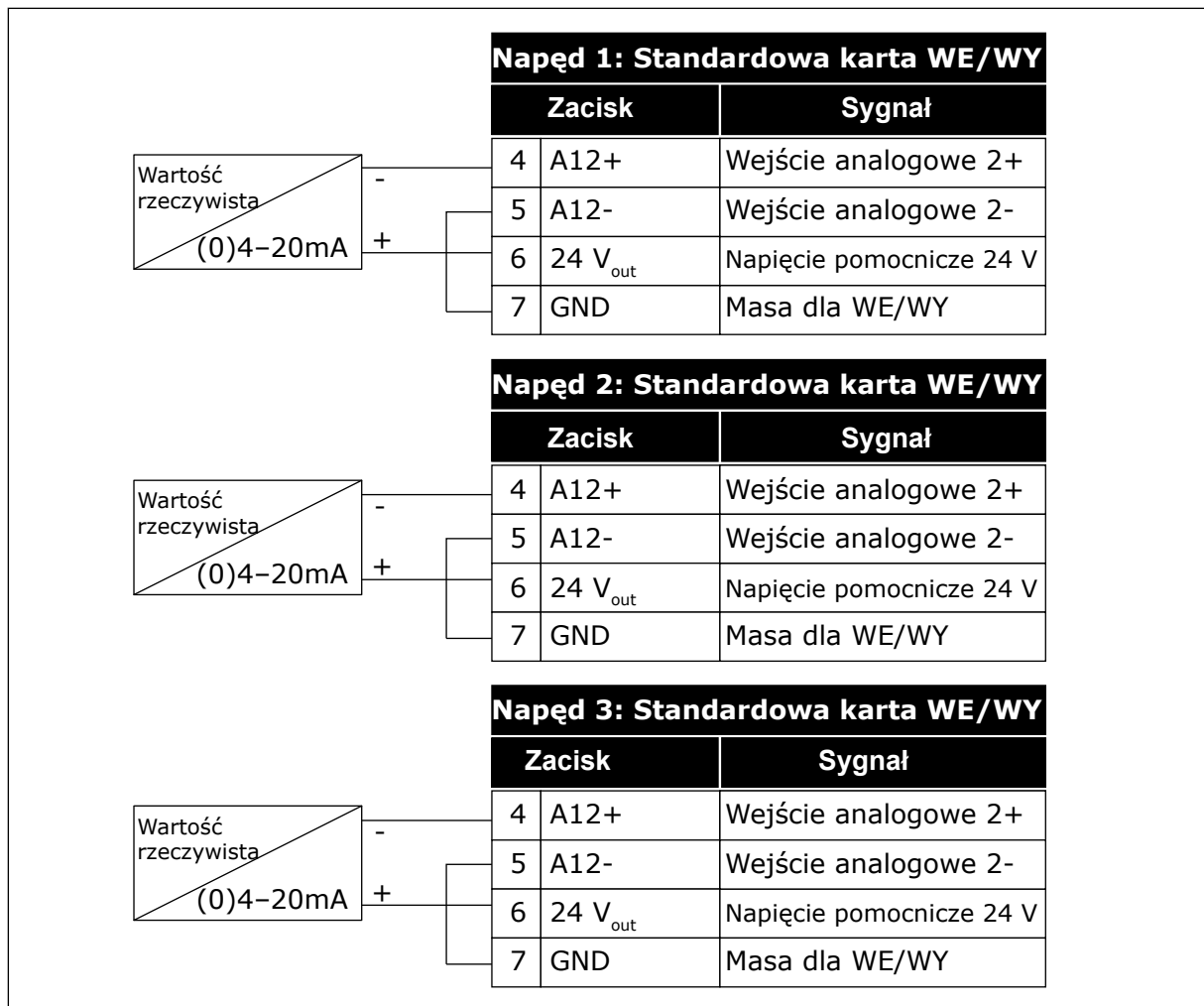
Rys. 94: Okablowanie czujników sprzężenia zwrotnego dla każdego napędu
