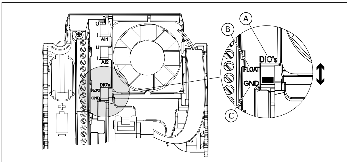
Rys. 97: Przetłącznik DIP izolacji
