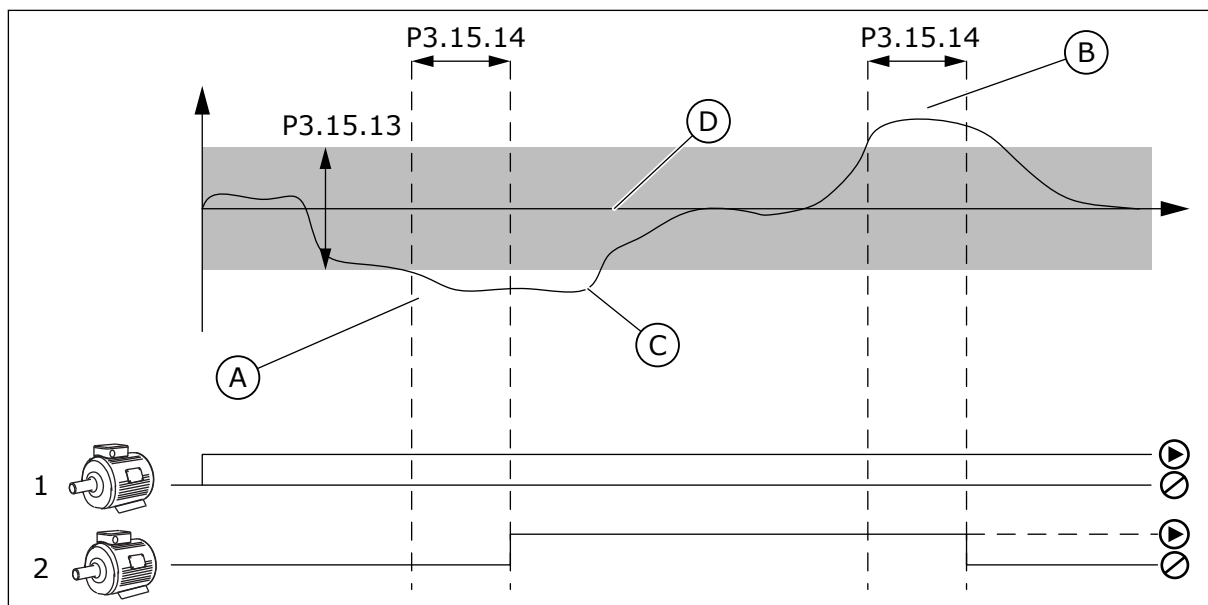
Rys. 99: Uruchamianie lub zatrzymanie pomp pomocniczych (P3.15.13 = szerokość pasma, P3.15.14 = opóźnienie szerokości pasma)
