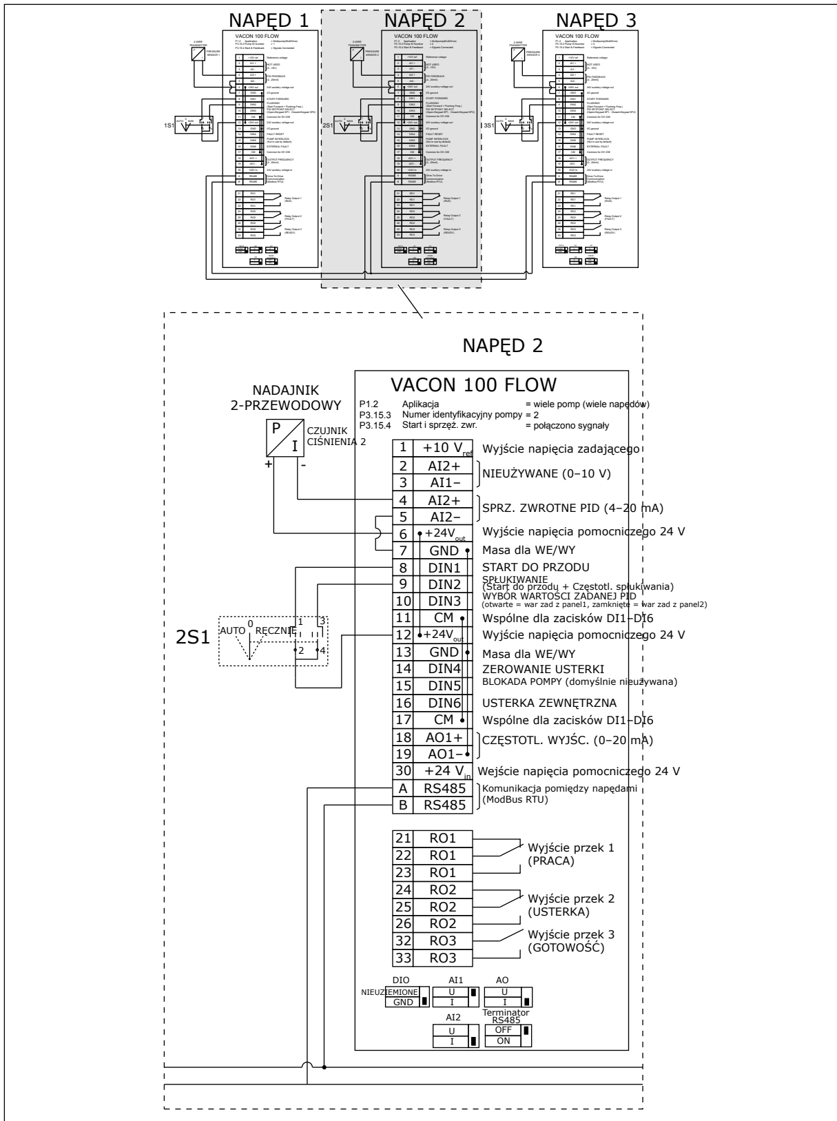
Rys. 19: Schemat połączeń elektrycznych w systemie wielonapędowym (wielonapędowym), przykład 1B
